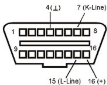
Диагностический разъем OBD-II в а/м Renault
